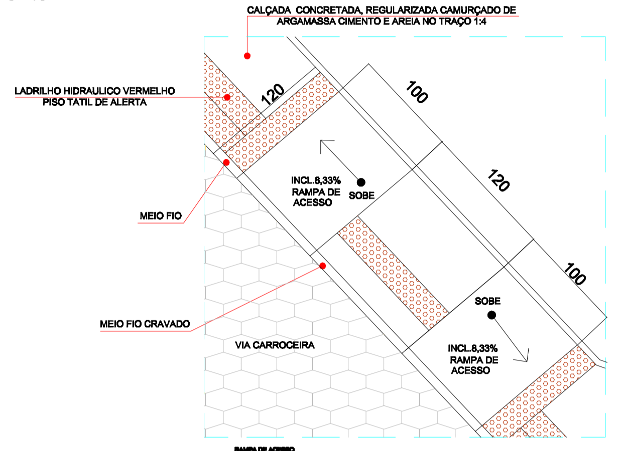
DETALHE 02 ESC.: 1/60
