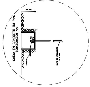
DETALHE ATERRAMENTO
