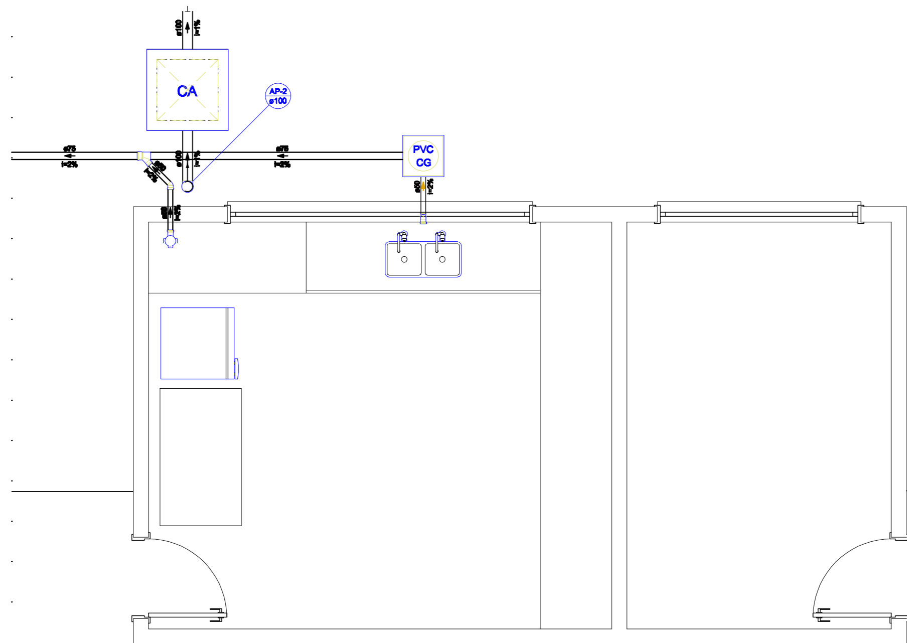
Térreo - Sanitário DETALHE SAN 1 1:25
